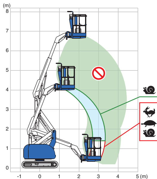
Werkbereik AA-9MC
